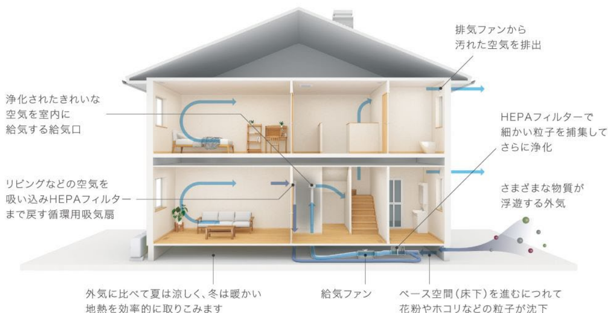
※エコナビ搭載換気システムHEPA+(プラス)の空気の流れのイメージ図です。 ※住宅の仕様により、換気システムは変更する場合があります。
