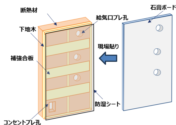
外壁パネル室内側の内装部 イメージ
