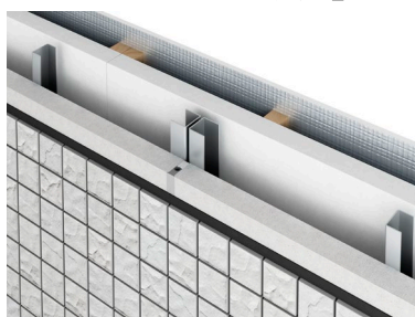
断熱材:ポリスチレンフォーム
