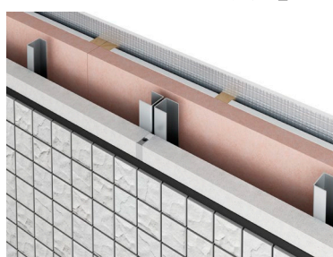
断熱材:フェノールフォーム+ポリスチレンフォーム
