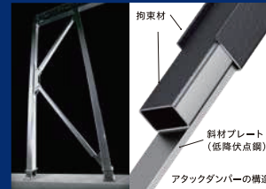
先進技術を採用した高耐力制震フレーム
