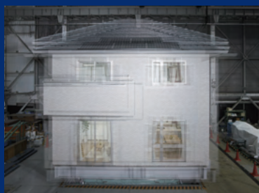
実験施設の限界に挑戦した耐震実験
